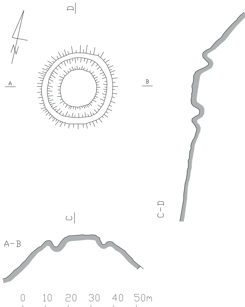
Sl. 1 Skica kasnosrednjovjekovnog visinskoga gradišta Lepavina – Gradina (crtež: T. Tkalčec) Fig. 1 Sketch of the late medieval Lepavina – Gradina hillfort (drawing by: T. Tkalčec)
