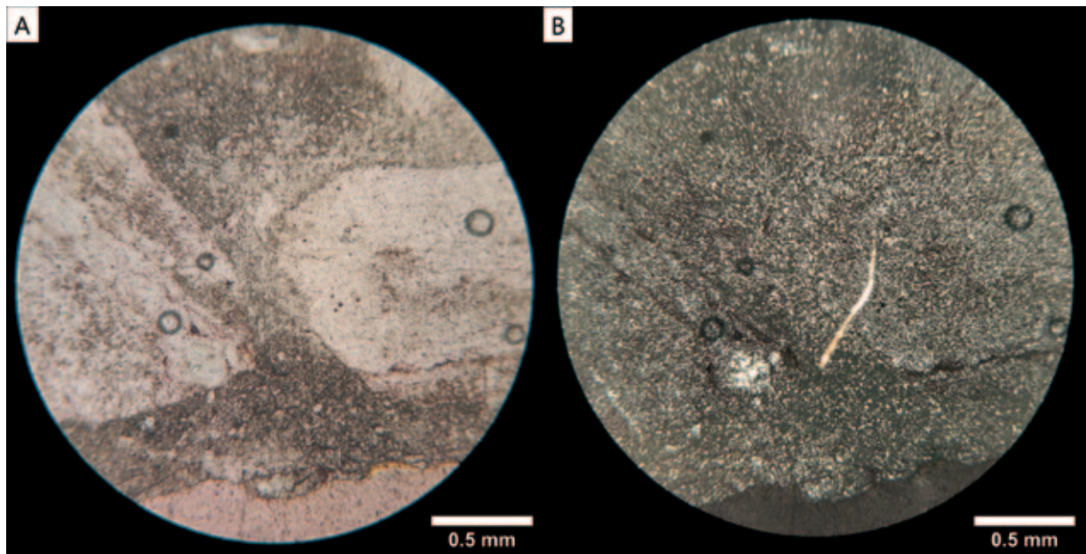
Sl. 28 Jedan od uzoraka rožnjaka iz uvale Polje. Djelomično zaobljeni litoklasti niske sferičnosti: A povećanje 40x, polarizirano svjetlo; B povećanje 40x, ukriženi nikoli (izradila: K. Šprem) Fig. 28 One of the chert samples from Polje Bay. Sub-rounded lithoclasts of low sphericity: A magnification 40x, polarized light; B magnification 40x, crossed polars (made by: K. Šprem)
