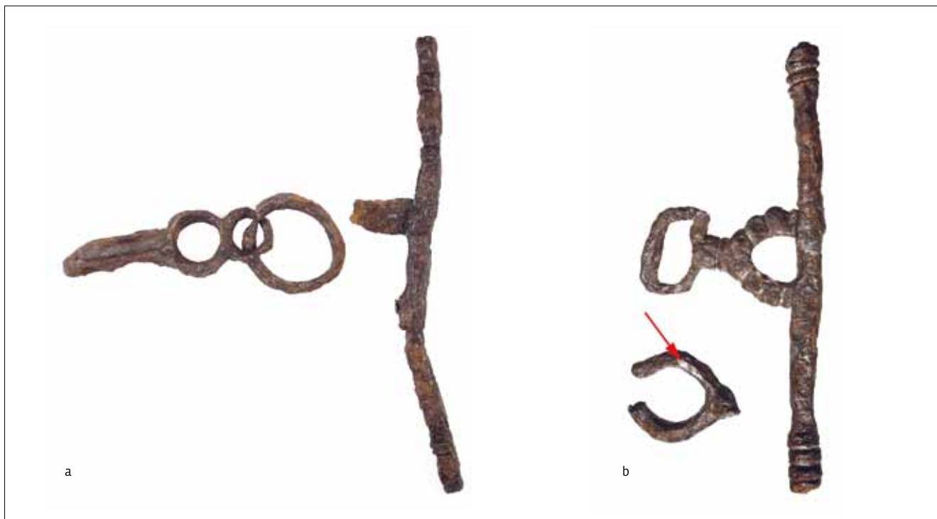
SLIKA 4. Dijelovi većih (a) i manjih (b) žvala s označenim mjestom na kojem je provedena analiza i EDS spektar (c) s jasno vidljivim linijama olova i kositra (snimio i izradio D. Doračić).
