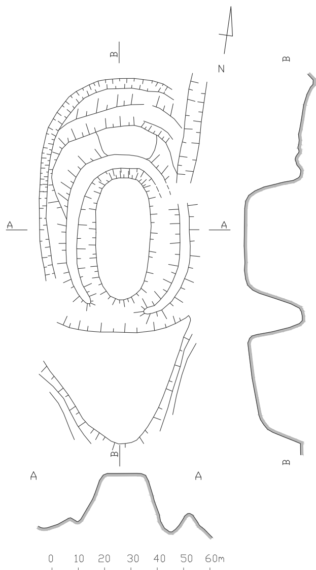
Sl. 2 Rasinja-Opoj grad, tlocrt i presjeci (crtež: T. Tkalčec) Fig. 2 Rasinja – Opoj-grad, layout and cross-sections (drawing: T. Tkalčec)
