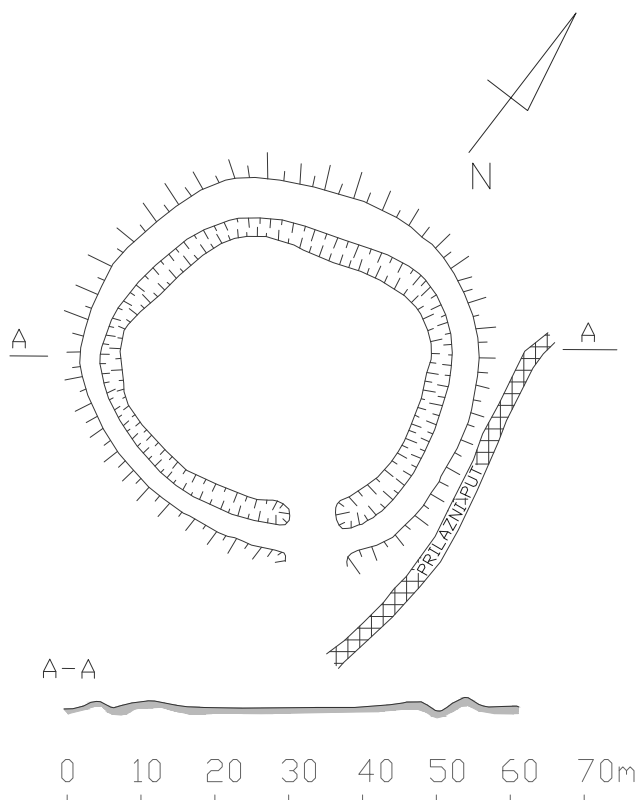
Sl. 9 Veliki Poganac – Šanac, tlocrt i presjek (crtež: T. Tkalčec)
