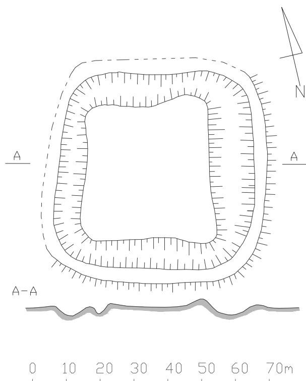
Sl. 7 Veliki Poganac – Gradina, tlocrt i presjek (crtež: T. Tkalčec)
