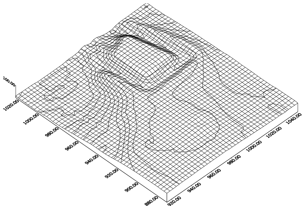
Sl. 11 Osijek Vojakovački – Mihalj, tlocrt, 3D ortogonalna projekcija (snimak i obrada: T. Tkalčec)
