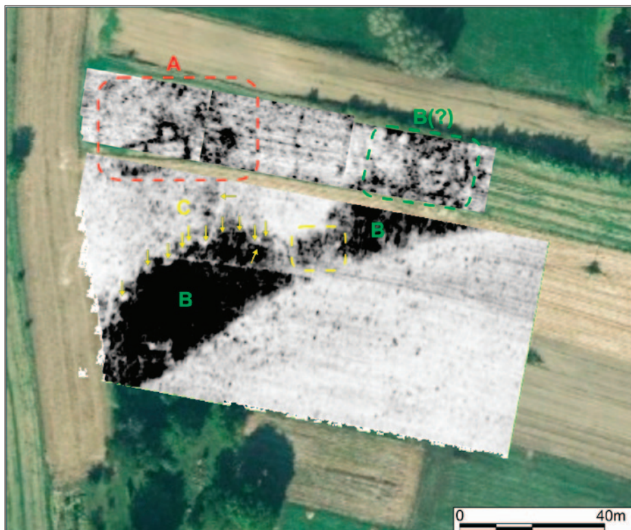
Sl. 3 Rezultati georadarske metode primjenom 400 MHz antene (izradió: B. Mušić)
