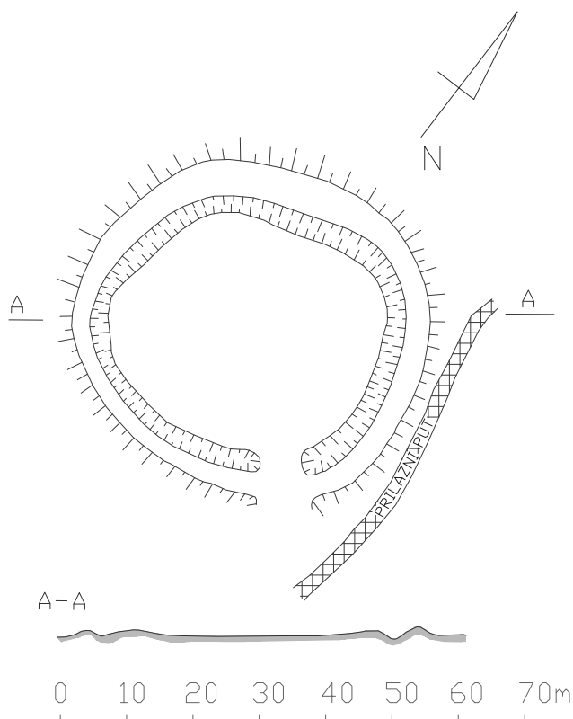
Sl. 9 Veliki Poganac – Šanac, tlocrt i presjek (crtež: T. Tkalčec)
