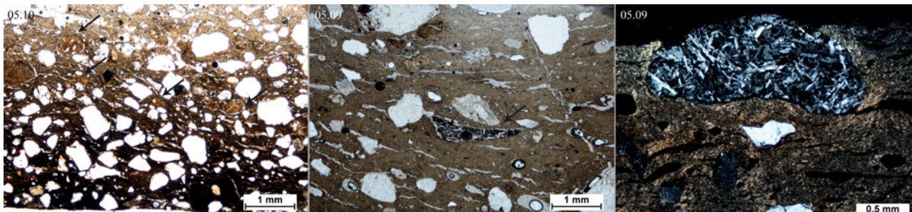
Sl. 6 Mikrofotografije uzoraka keramike: glinoviti peleti u matrici (05.10.), biljni materijal u praznini (05.09.), krupne primjese stijena (05.09) (izradila: A. Kudelić) Fig. 6 Photomicrographs of pottery samples: clay pellets in a matrix (05.10.), plant material in a void (05.09.), large rock temper (05.09) (made by: A. Kudelić)
