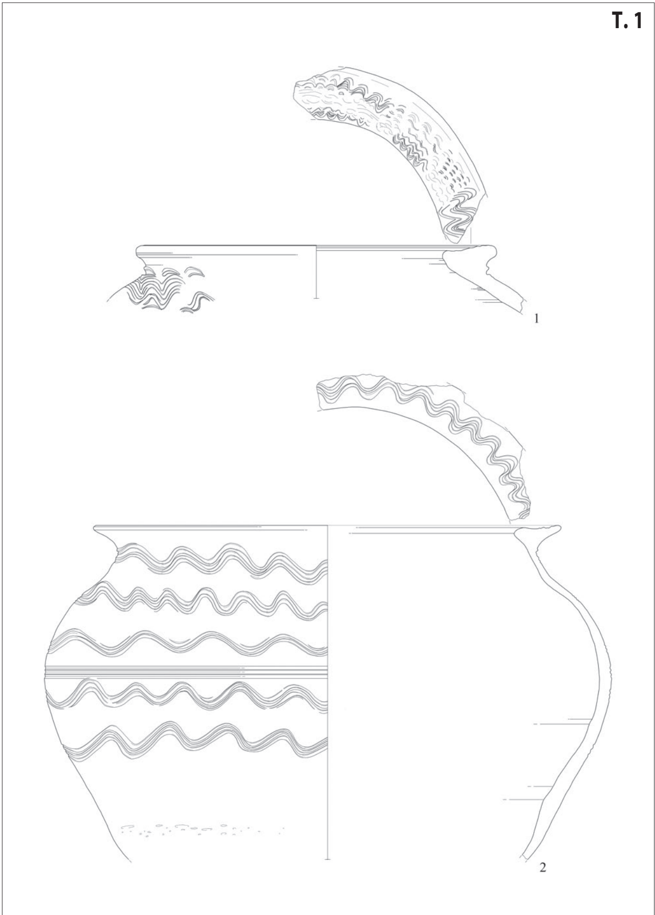
T. 1 Rifnik: kasnorimski lonci za pohranu (crtež: M. Bausovac; M 1:3)
