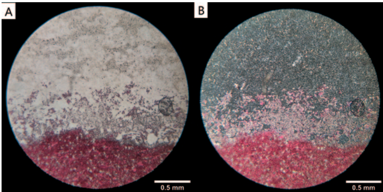
Sl. 16 Izbrusak rožnjaka pronađenog u Poljakima, povećanje 40x: A polarizirano svjetlo; B ukriženi nikoli (izradila: K. Šprem; Šprem 2022: 43, mikrofotografija 7) Fig. 16 Thin section of a chert sample from Poljaki, magnification 40x: A polarized light; B crossed polars (made by: K. Šprem; Šprem 2022: 43, microphotography 7)
