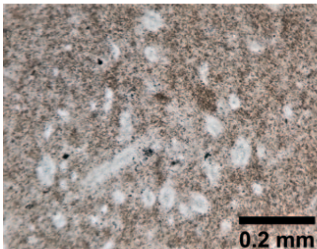
Sl. 21 Duhovi mikrofosila u kriptokristalnoj kvarcnoj masi onečišćenju limonitom. Povećanje 100x, polarizirano svjetlo (izradila: K. Šprem; Šprem 2022: 48, mikrofotografija 9)
