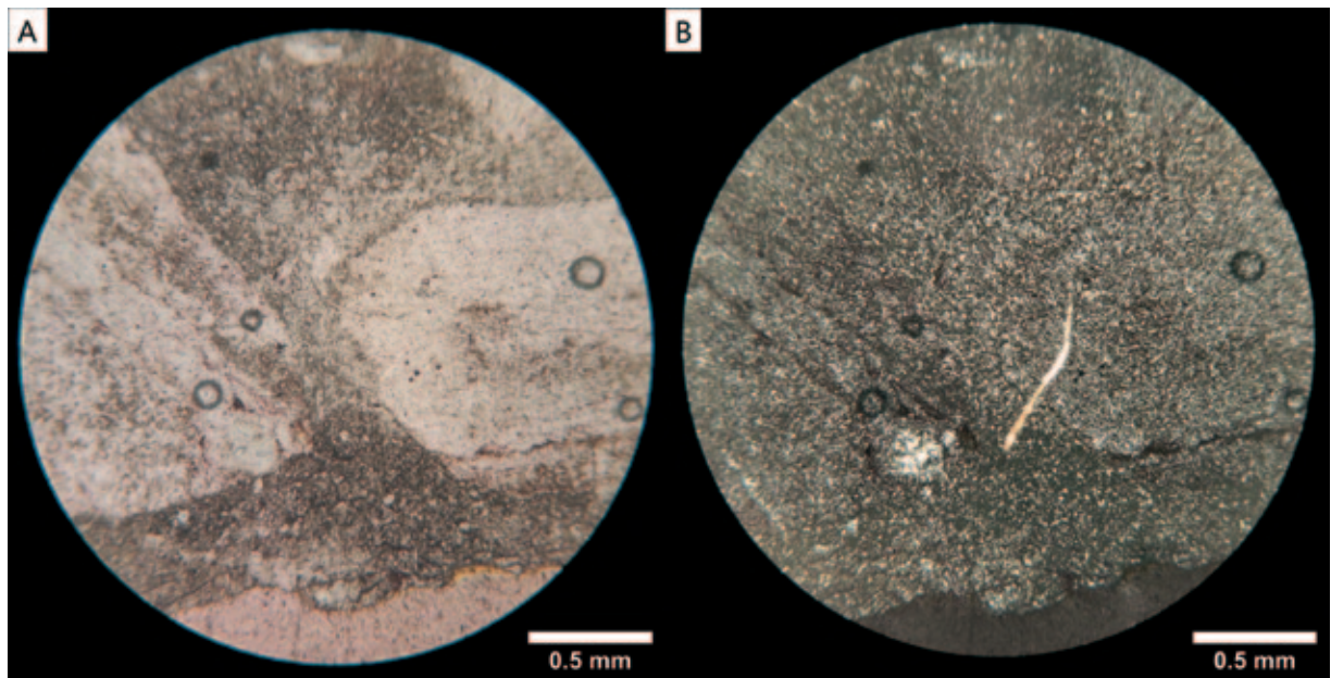
Sl. 28 Jedan od uzoraka rožnjaka iz uvale Polje. Djelomično zaobljeni litoklasti niske sferičnosti: A povećanje 40x, polarizirano svjetlo; B povećanje 40x, ukriženi nikoli (izradila: K. Šprem)
