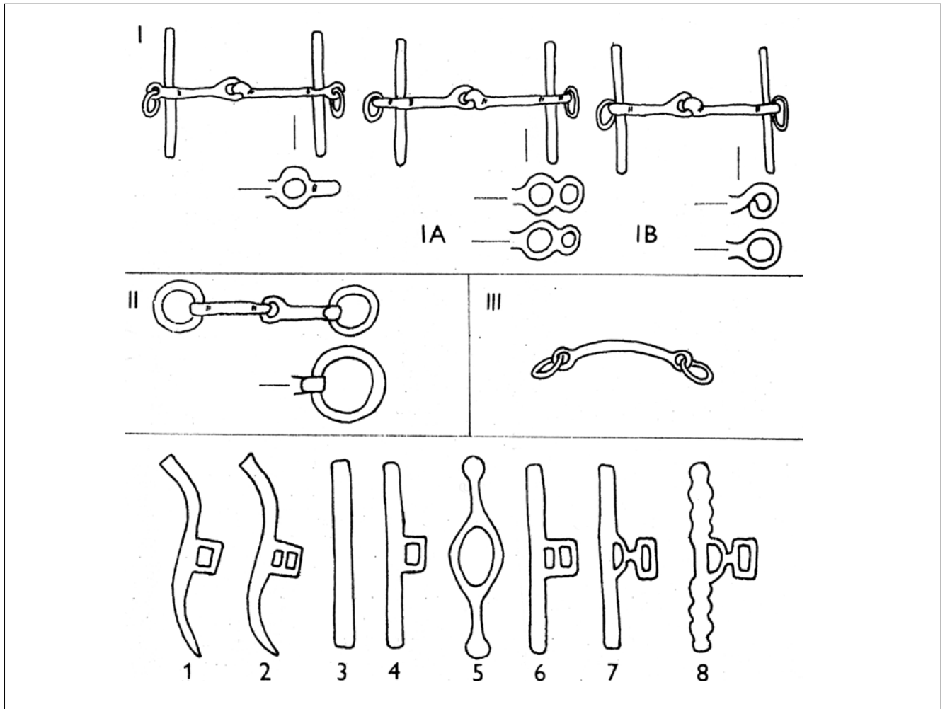
FIGURE 5. The typology of bits according to Měchurová (Měchurová 1984, 267, Pl. I).
