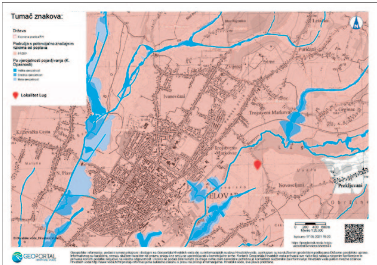
Karta 3 Položaj lokaliteta Lug u odnosu na grad Bjelovar i moguća okolna plavna područja (izvor: Geoportala Hrvatske vode; prilagodio: J. Drpić)
